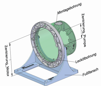
Einbaurichtung PTF5
