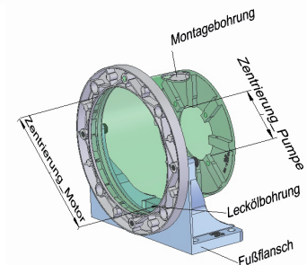
Einbaurichtung PTFL
